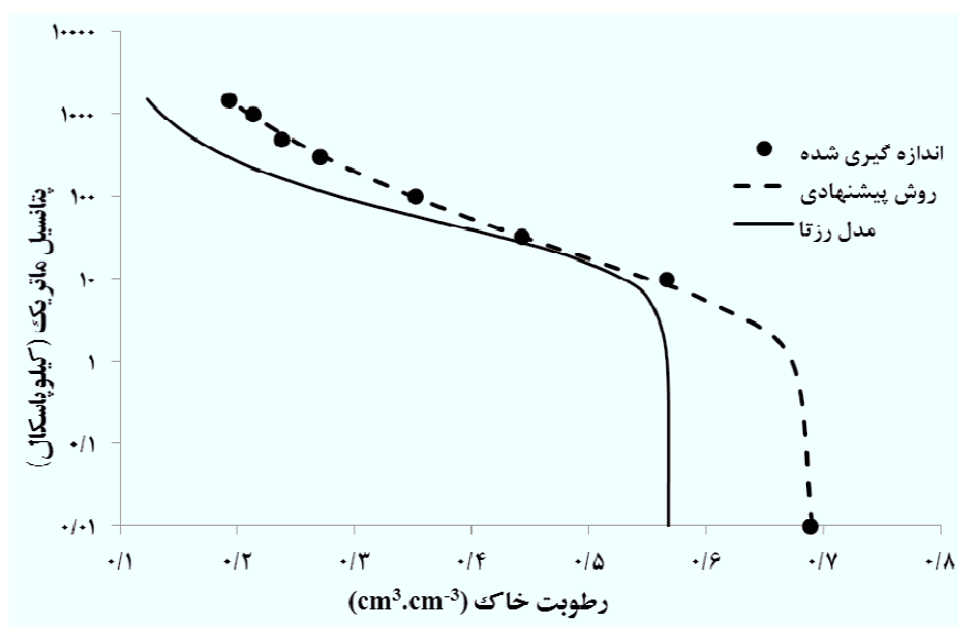
شکل ۳- نمونه‌ای از منحنی مشخصه اندازه‌گیری و پیش‌بینی شده به وسیله دو روش (نمونه شماره ۵۹ از بانک اطلاعاتی خالق‌پناه)
