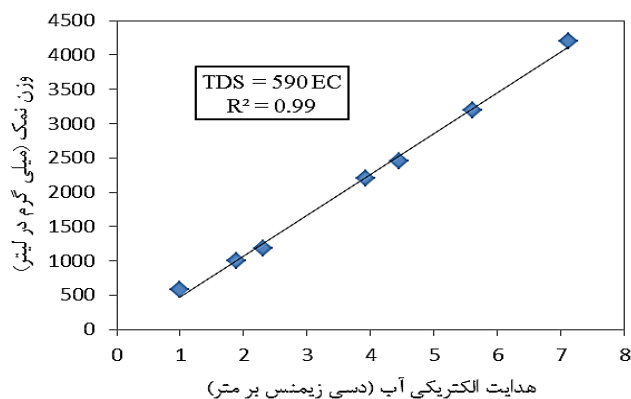
شکل ۱- نمودار کالیبراسیون هدایت الکتریکی آب با نمک
