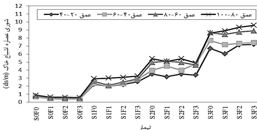
شکل ۵- شوری عصاره اشباع در نیمرخ خاک، تحت تأثیر تیمارها
