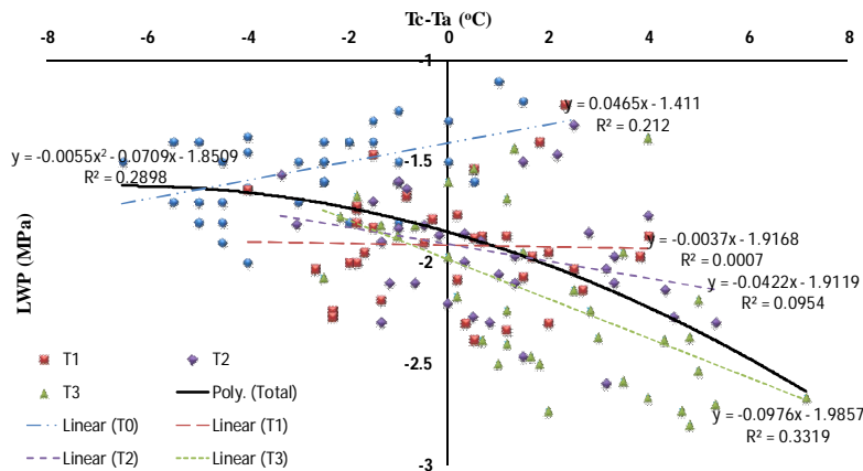
شکل 7- ارتباط پتانسیل آب برگ و اختلاف دمای تاج درخت با هوا
