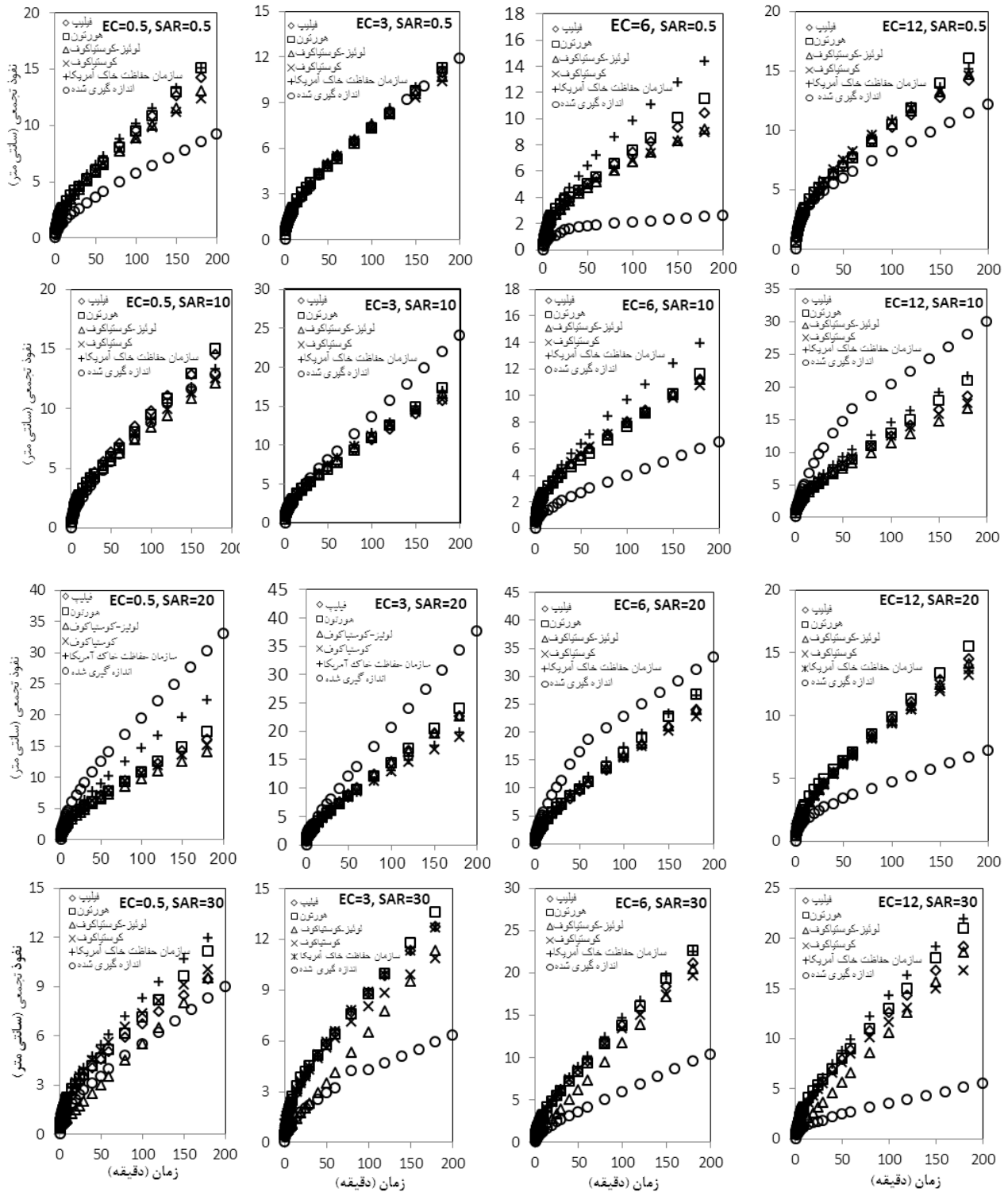
شکل ۱ - مقایسه نفوذ تجمعی (سنتی متر) اندازه‌گیری و برآورد شده با مدل‌های نفوذ با گذشت زمان (دقیقه) برای نفوذ آب‌های با قابلیت هدایت الکتریکی ( EC, dS m^{-1} ) و نسبت جذب سدیم ( SAR, meq^{0.5} L^{0.5} ) متفاوت در خاک سری دانشکده
