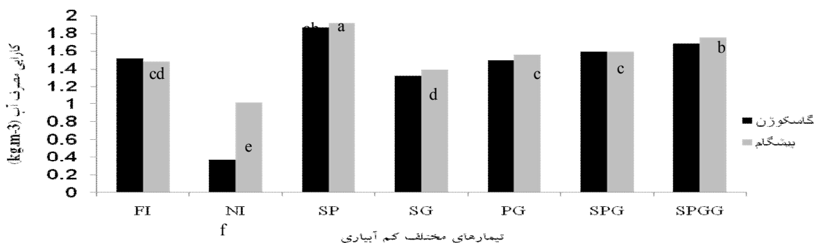
شکل ۲. تغییرات کارایی مصرف آب زئوتیپ‌های مقاوم (بیشگام) و حساس (گاسکوژن) به خشکی تحت تیمارهای مختلف کم آبیاری
